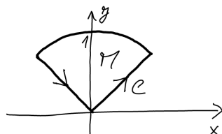
Obrázek 6: Množina M a křivka C .
